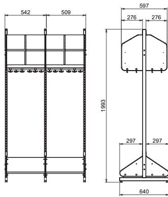
BST typ B, två platser (med platsbredd 250 mm)
