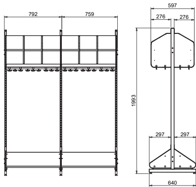
BST typ B, tre platser (med platsbredd 250 mm)
