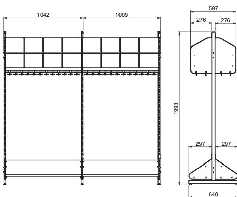
BST typ B, fyra platser (med platsbredd 250 mm)
