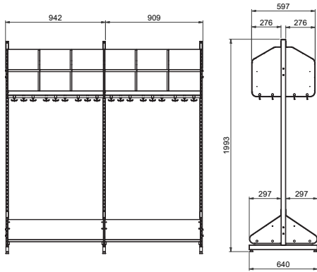
BST typ B, tre platser (med platsbredd 300 mm)
