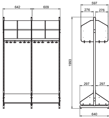
BST typ B, tre platser (med platsbredd 300 mm)
